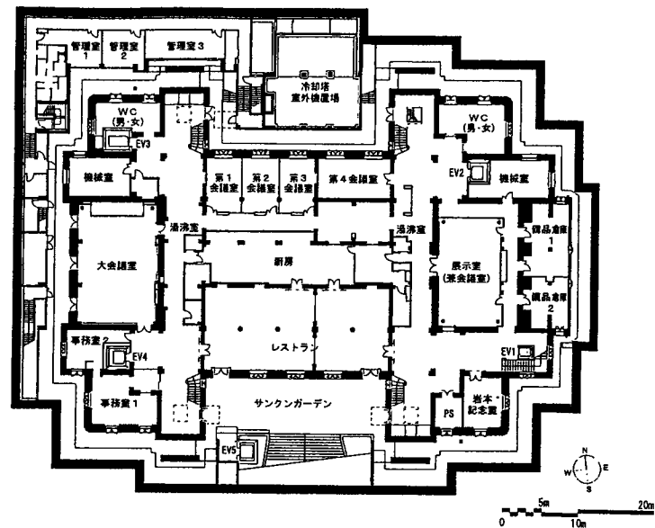
地階平面図
