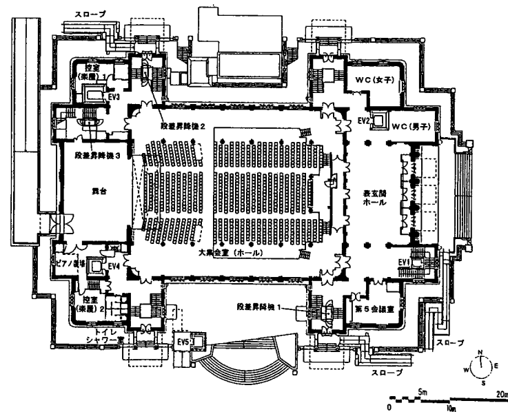
1階平面図
